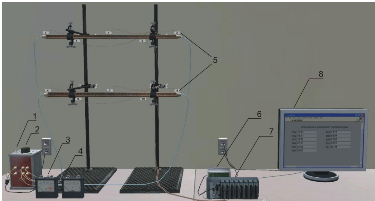
Рис. 3.3. Схема экспериментальной установки
